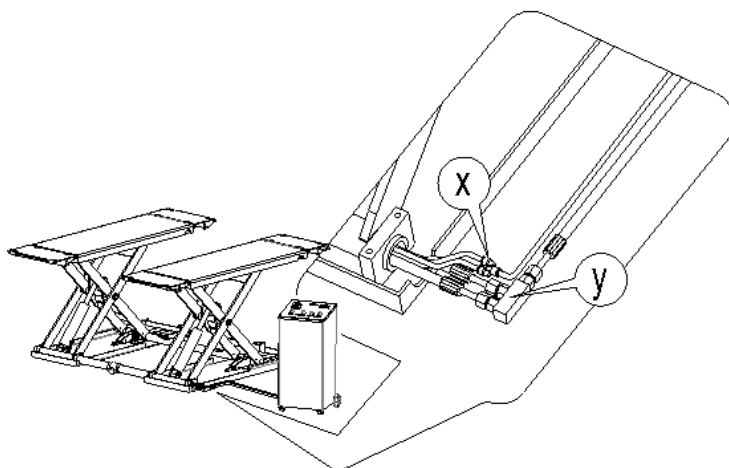
Rysunek 8. Przewody hydrauliczne i elektryczne
