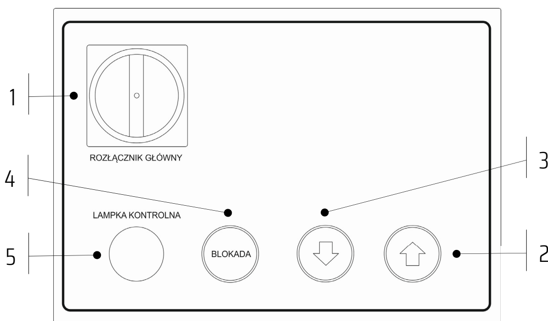
Rysunek 10. Panel sterujący
