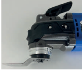
Posuňte páčku dozadu, odomknite dvojitú poistku.
